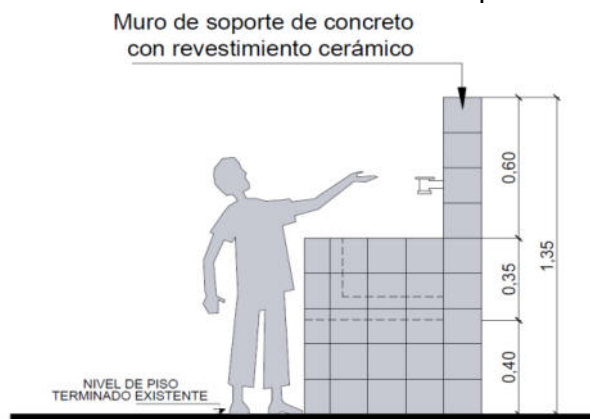
Gráfico N° 4. Lavadero lineal nivel primaria
